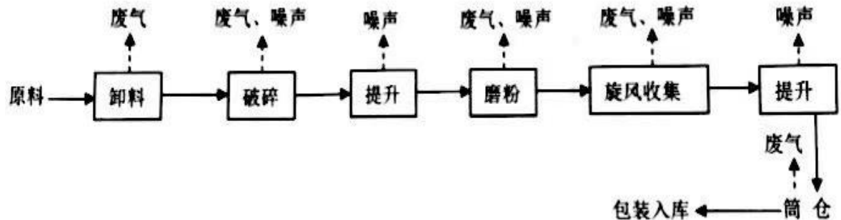
图 4-1 生产工艺流程图及排污节点
