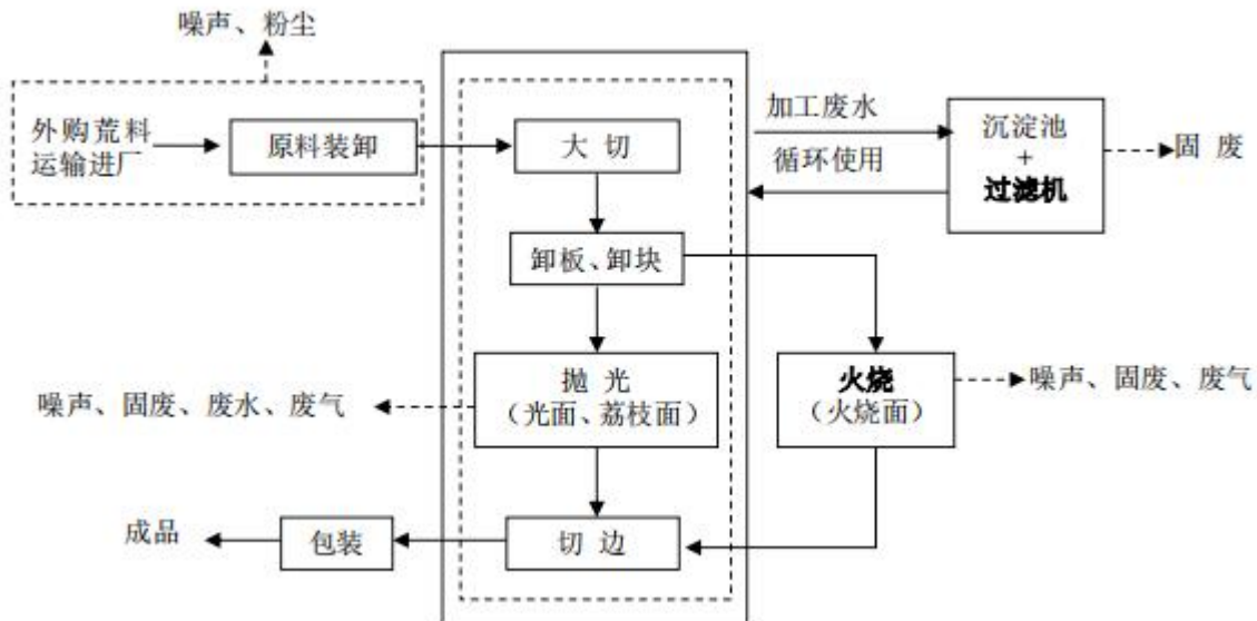
图 4-1 生产工艺流程图及排污节点
